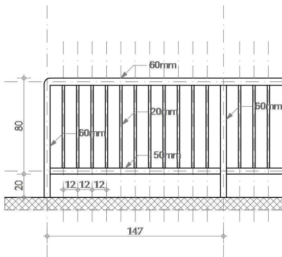
DETALJ OGRADE R 1:30
